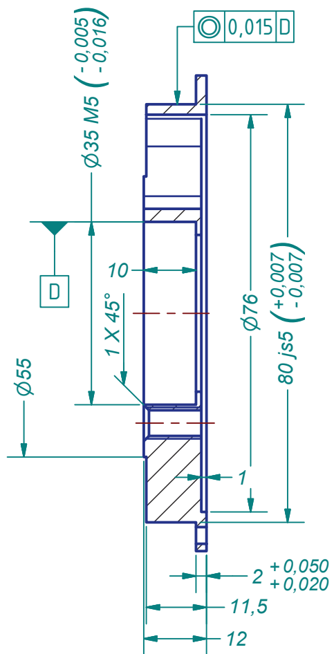
B-B ( 1 : 1 )
